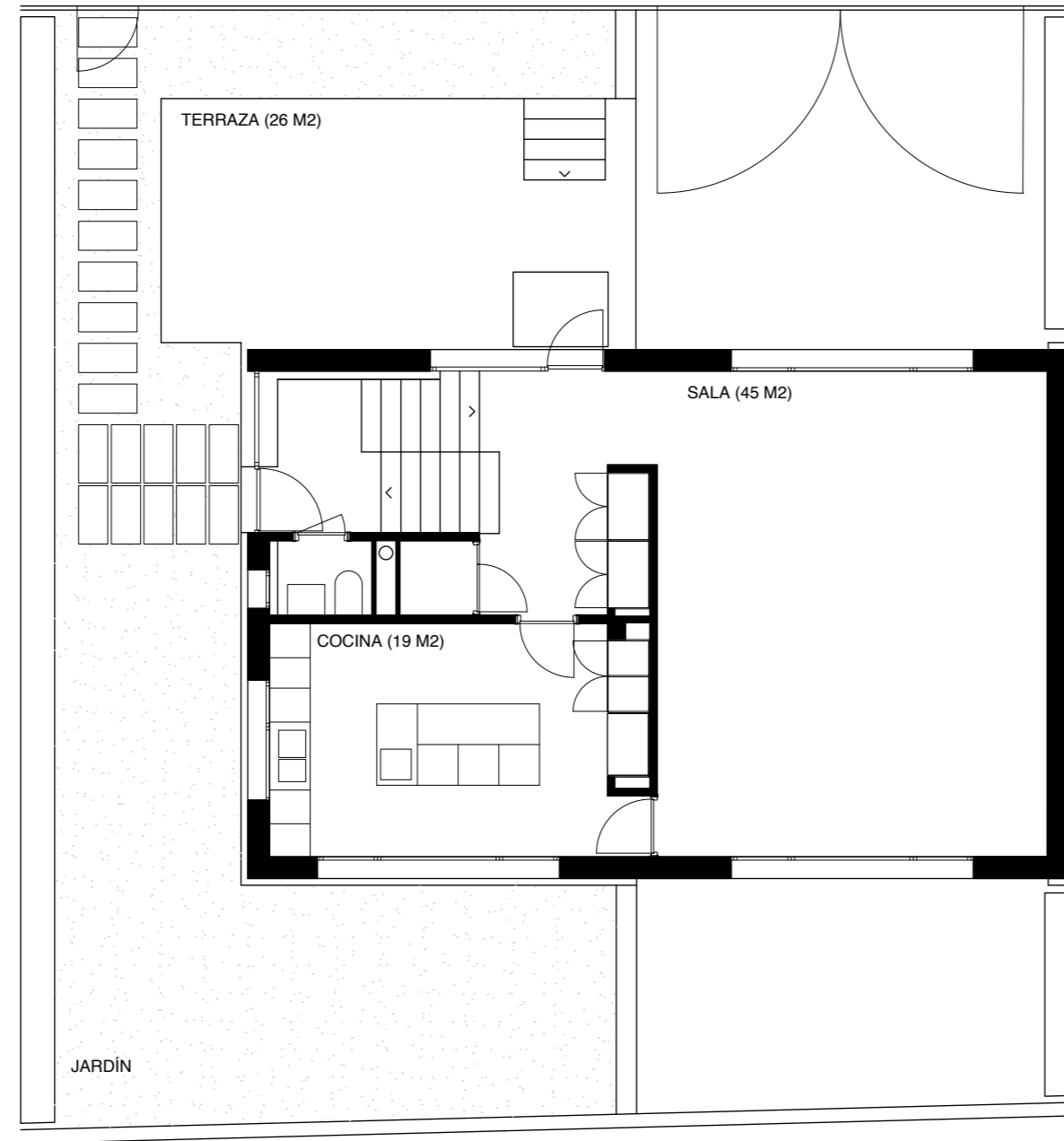
PLANTA BAJA
